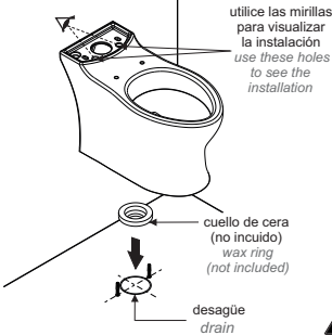
instalación con cuello de cera wax ring installation
