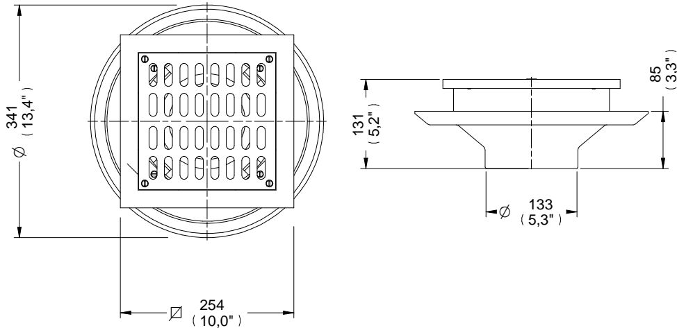
Medidas Referenciales/Estimated Dimensions, Acot.mm.(pulg)/Dim.mm.(in)
